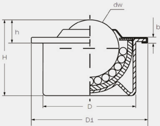
SPS 15-22-30
